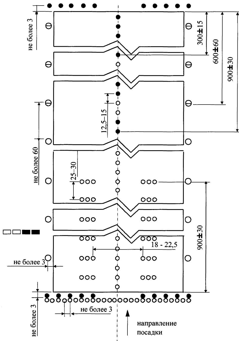
Рисунок 10. Схема расположения огней приближения систем ОВИ-II и ОВИ-III с интервалом 30 м (с дополнительными световыми горизонтами)
