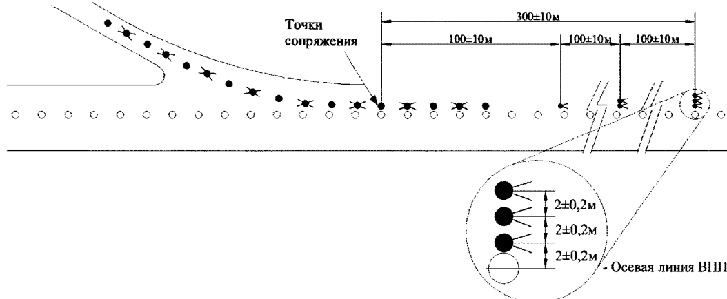
Рисунок 13. Огни указателя РД быстрого схода с ВПП
