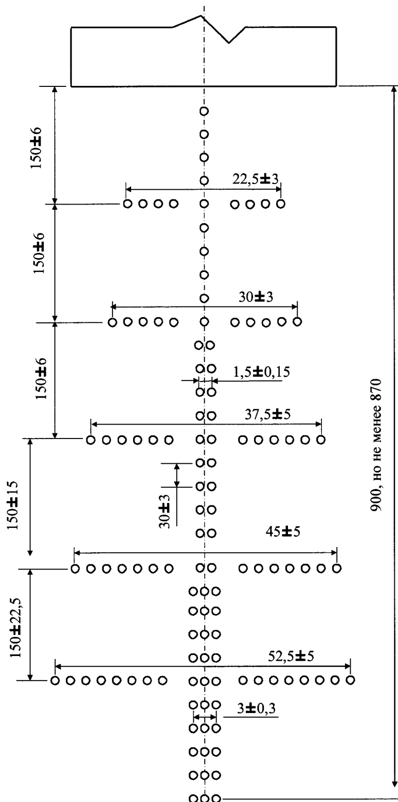
Рисунок 5. Схема расположения огней приближения системы ОВИ-I с интервалом 30 м (по центральному ряду)
