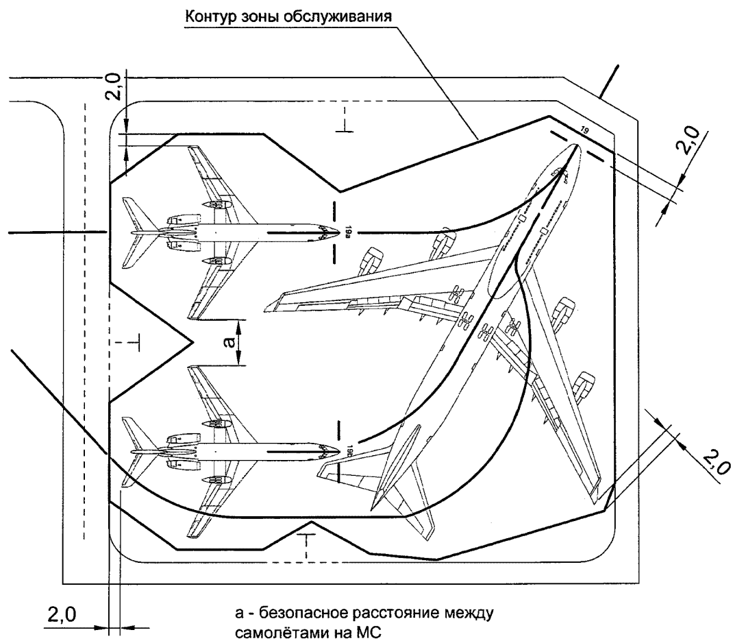
Рисунок 7. Схема маркировки перрона
