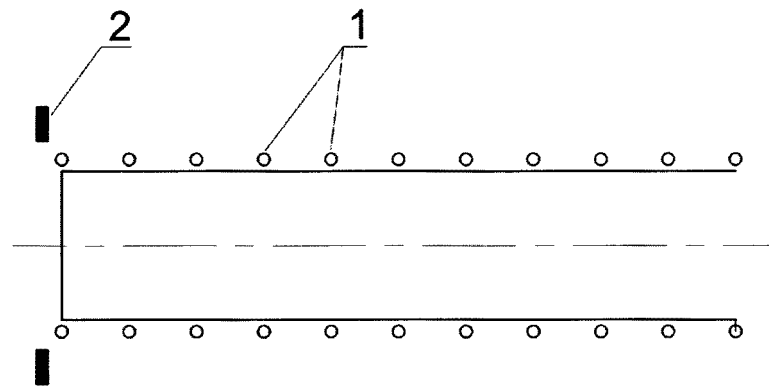
Рисунок 1. Схема оборудования ГВПП классов А, Б, В, Г, Д маркерами
