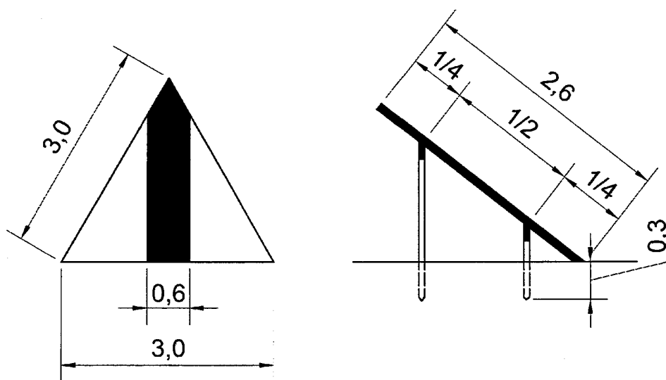
Осевой маркер между концом ЛП и БПРМ
