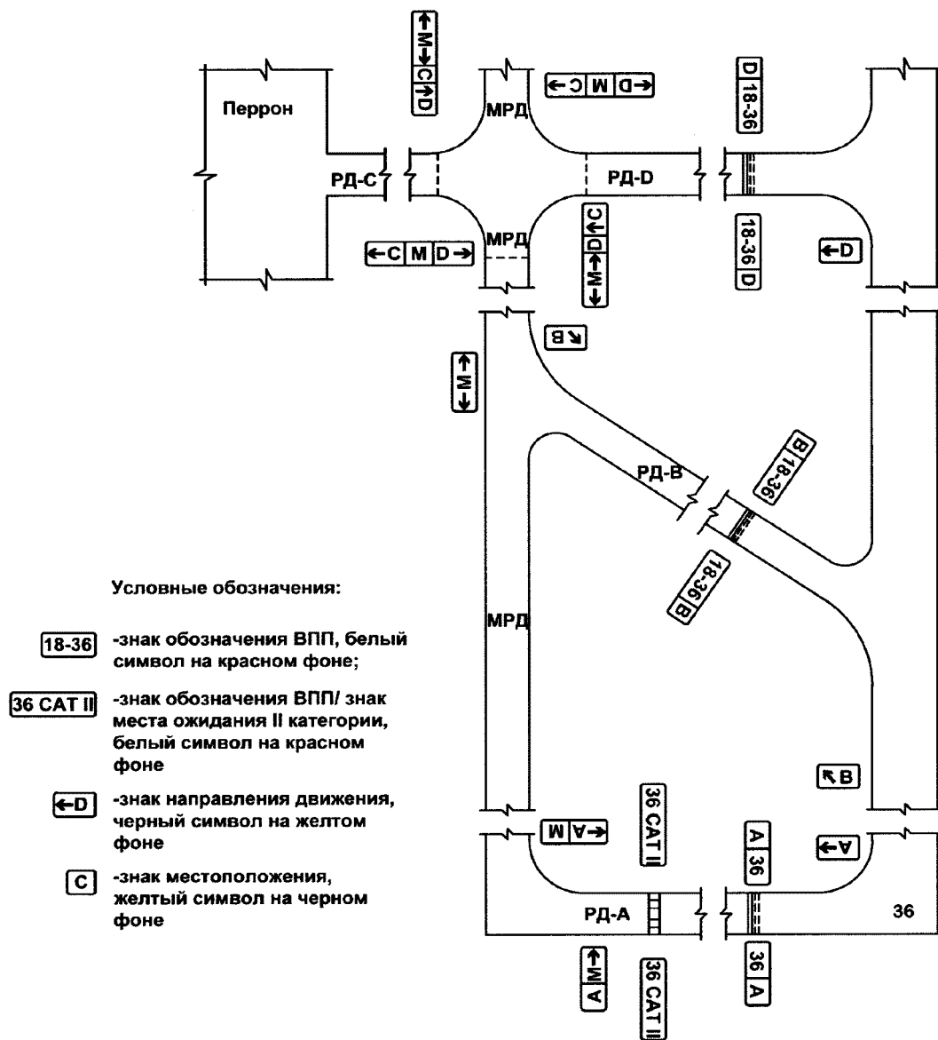
Рисунок 4. Пример расположения аэродромных знаков
