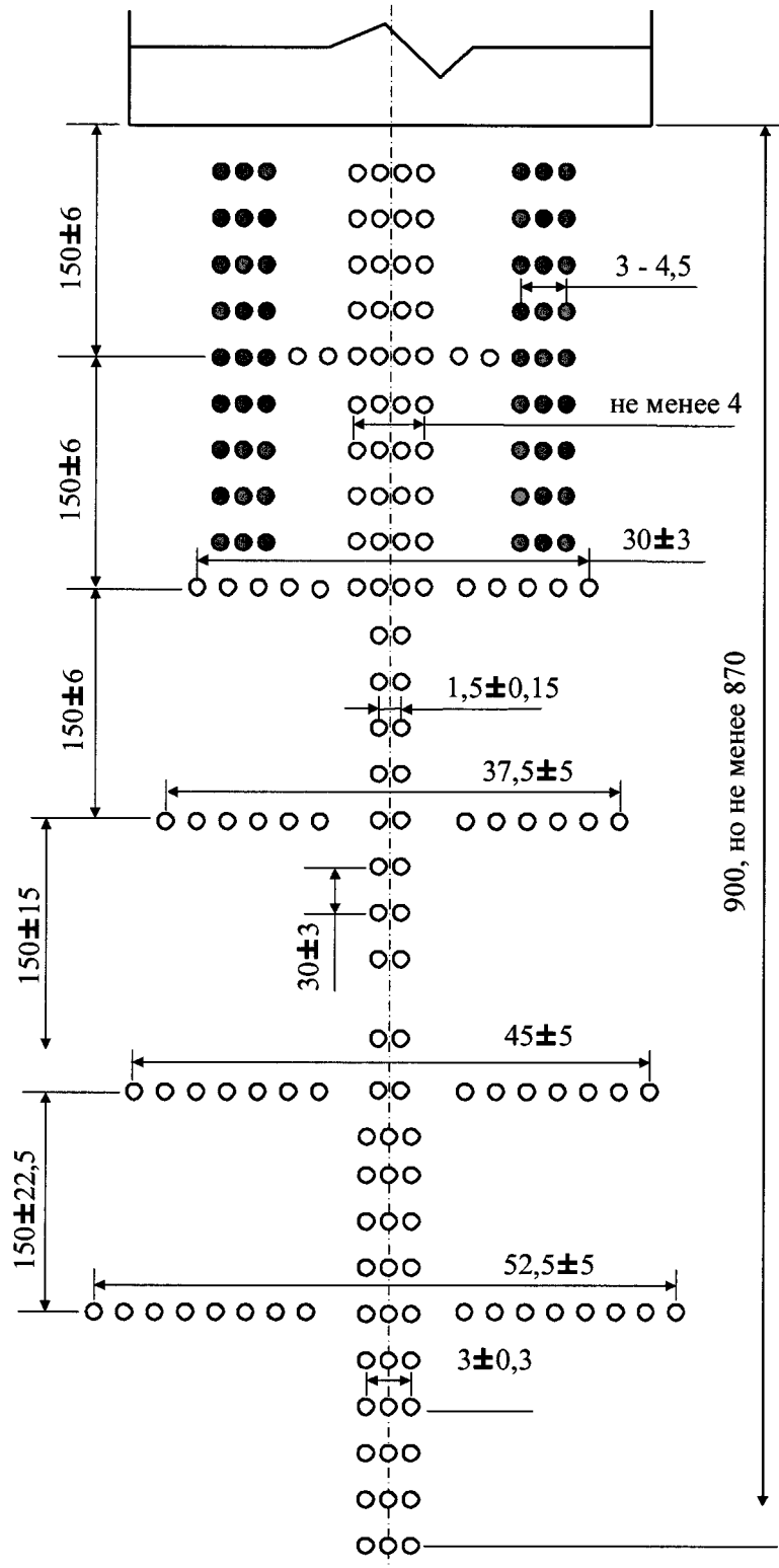
Рисунок 9. Схема расположения огней приближения системы ОВИ-II и ОВИ-III с интервалом 30 м
