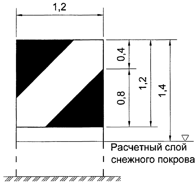
Рисунок 8. Маркер боковой границы
