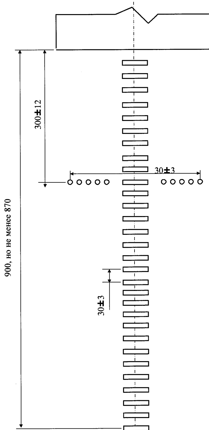
Рисунок 4. Схема расположения огней системы ОМИ при смещенном пороге ВПП
