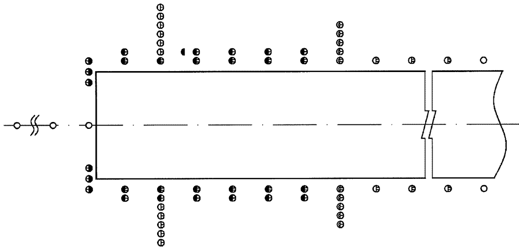
Рисунок 3. Схема расположения огней ВПП системы ОМИ
