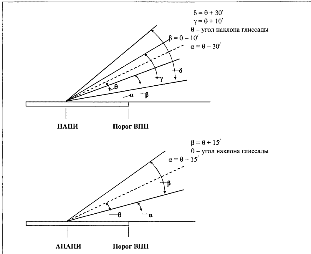
Рисунок 15. Углы возвышения огней в системах РАРИ и АРАРИ (для углов наклона глissады 2^\circ - 4^\circ )
