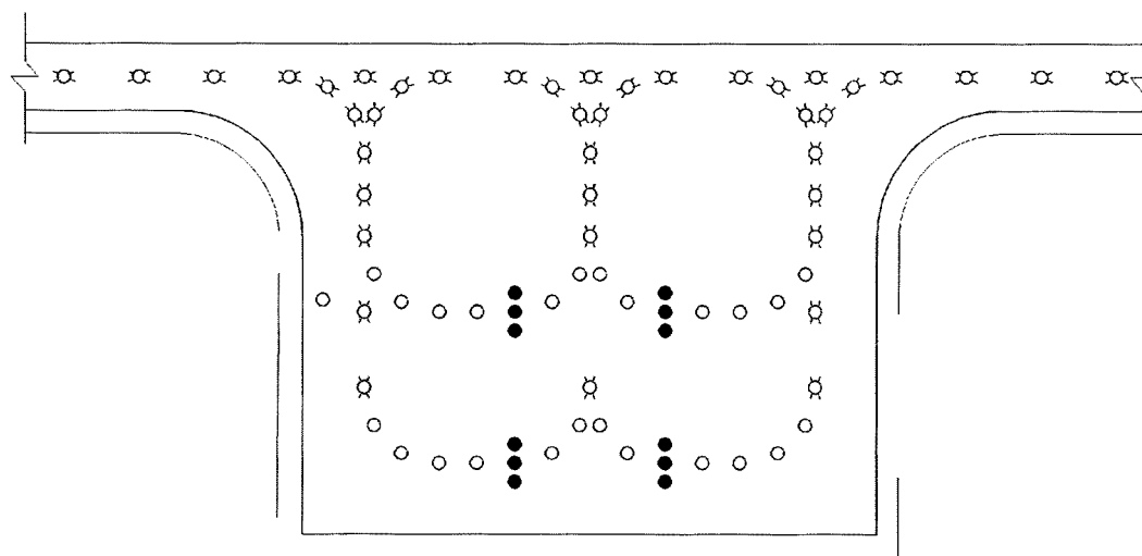
Рисунок 18. Огни защиты ВПП
