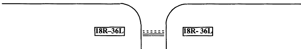
Рисунок 5. Примеры знаков обозначения ВПП в случае параллельных ВПП
