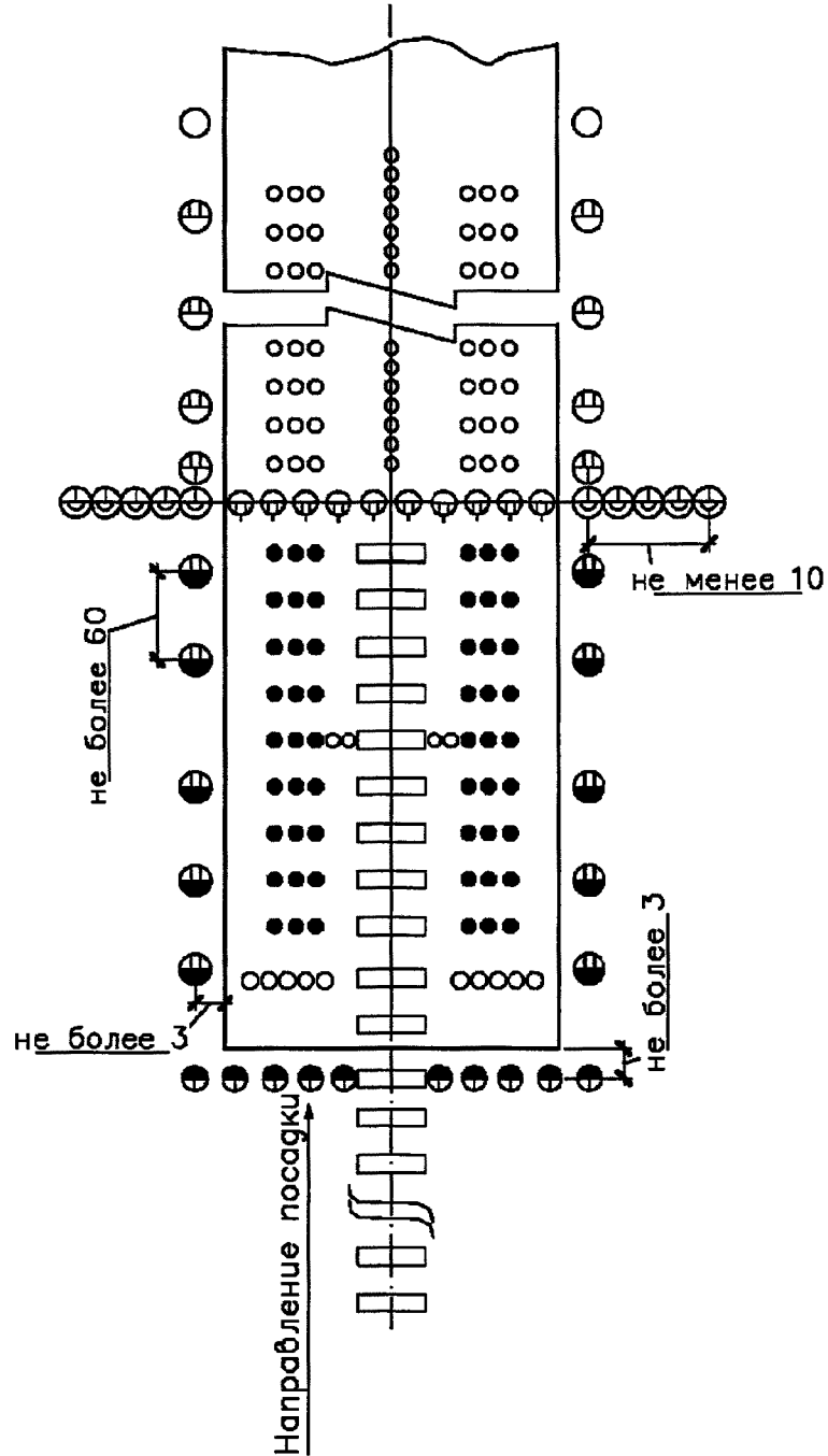
Рисунок 7. Схема расположения огней ВПП системы ОВИ-I с группами входных огней ВПП и системой РАРИ
