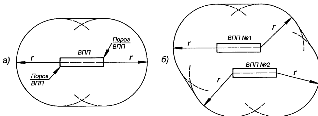
Рисунок 3. Внутренняя горизонтальная поверхность а) – для аэродрома с одной ВПП; б) – для аэродрома с двумя ВПП.
