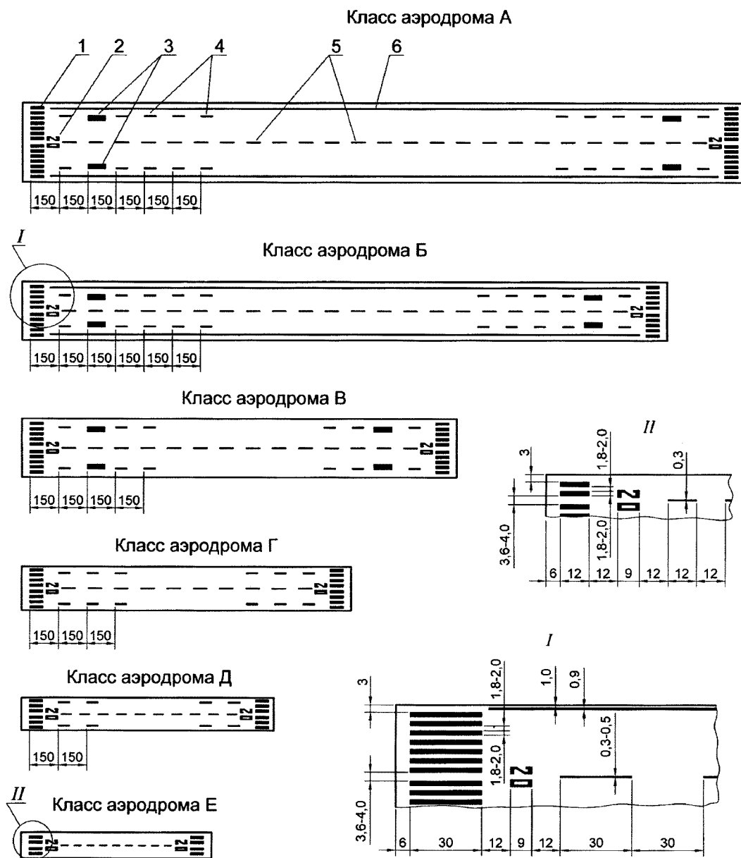
Рисунок 1. Схема маркировки аэродрома
