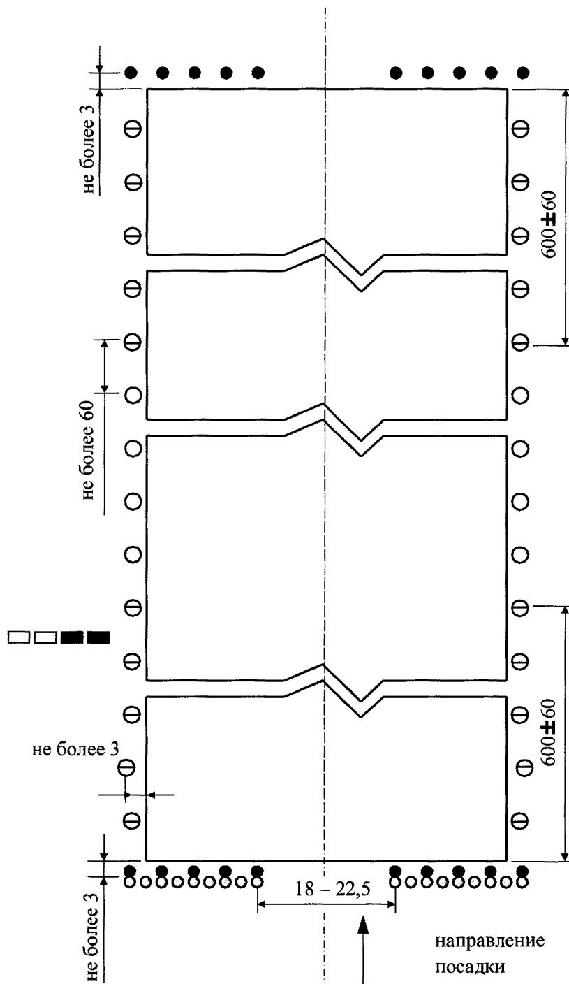
Рисунок 6. Схема расположения огней приближения системы ОВИ-I (с интервалом 30 м) с дополнительными световыми горизонтами
