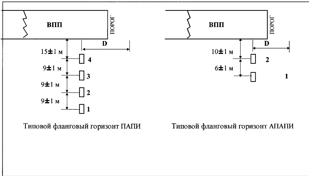
Рисунок 14. Расположение систем РАРИ и АРАРИ
