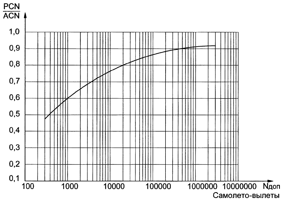
Зависимость допустимого количества самолето-вылетов типа ВС от соотношения PCN^{\#}/ACN^{\#}
