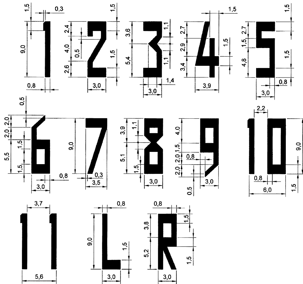
Рисунок 4. Размеры и форма цифр и букв на ИВПП
