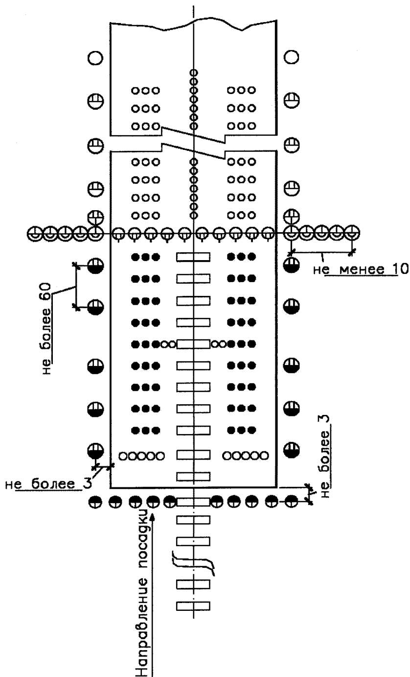
Рисунок 11. Схема расположения огней ВПП систем ОВИ-II и ОВИ-III с системой РАРИ с левой стороны ВПП
